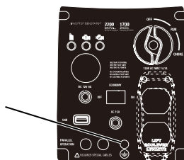
Figure 3-1. Mise à la terre du générateur
