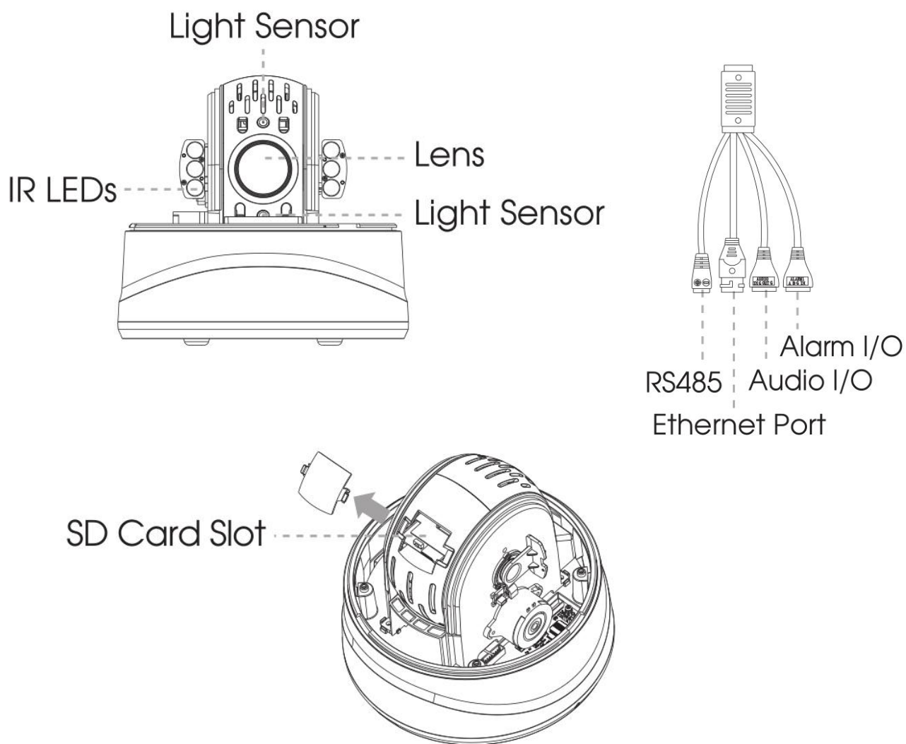
Figure 1-3-4 Mini PTZ Dome Network Camera
