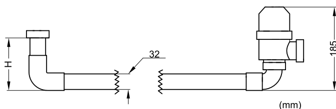
Рис. 7 Размеры и порядок сборки
