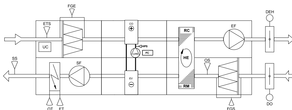
Рис. 10 Блок левого исполнения.
