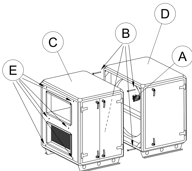
Рис. 5 Левосторонний агрегат
