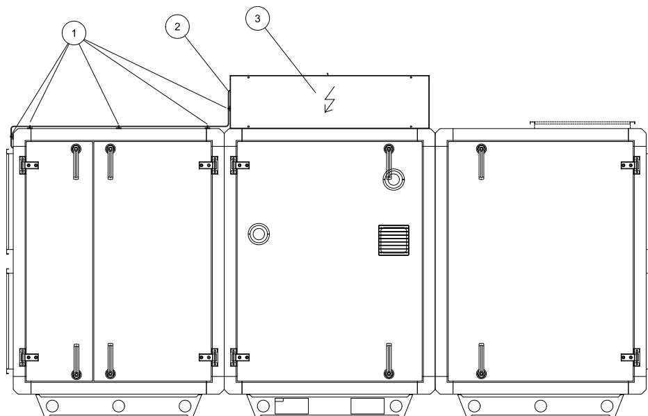
Рис. 9 Электрический монтаж, левосторонний агрегат
