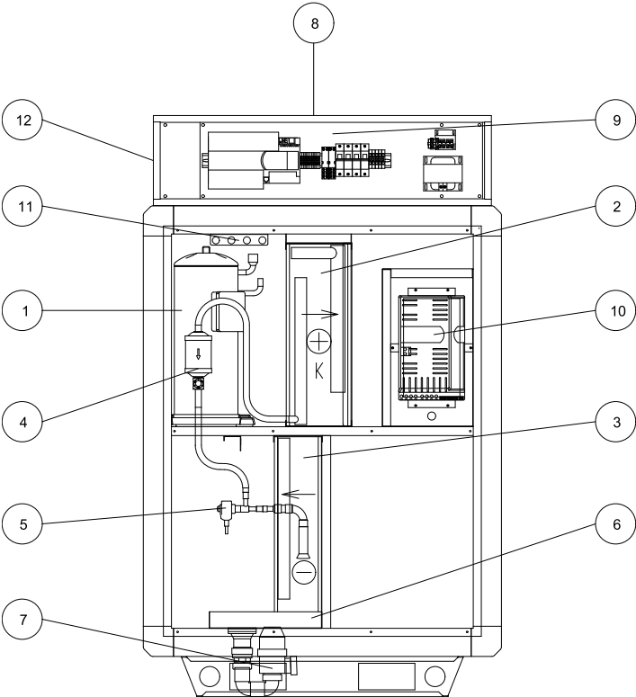
Рис. 2 Основные компоненты левостороннего агрегата
