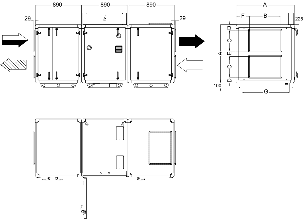
Рис. 1 Размеры SR09, SR11, мм (изображен левосторонний агрегат)
