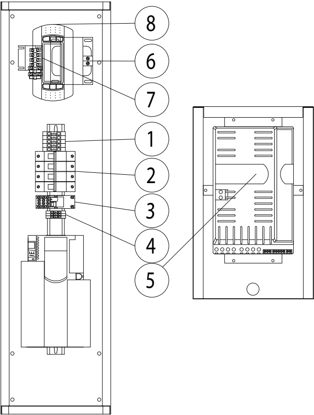
Рис. 3 Блок электрических подключений
