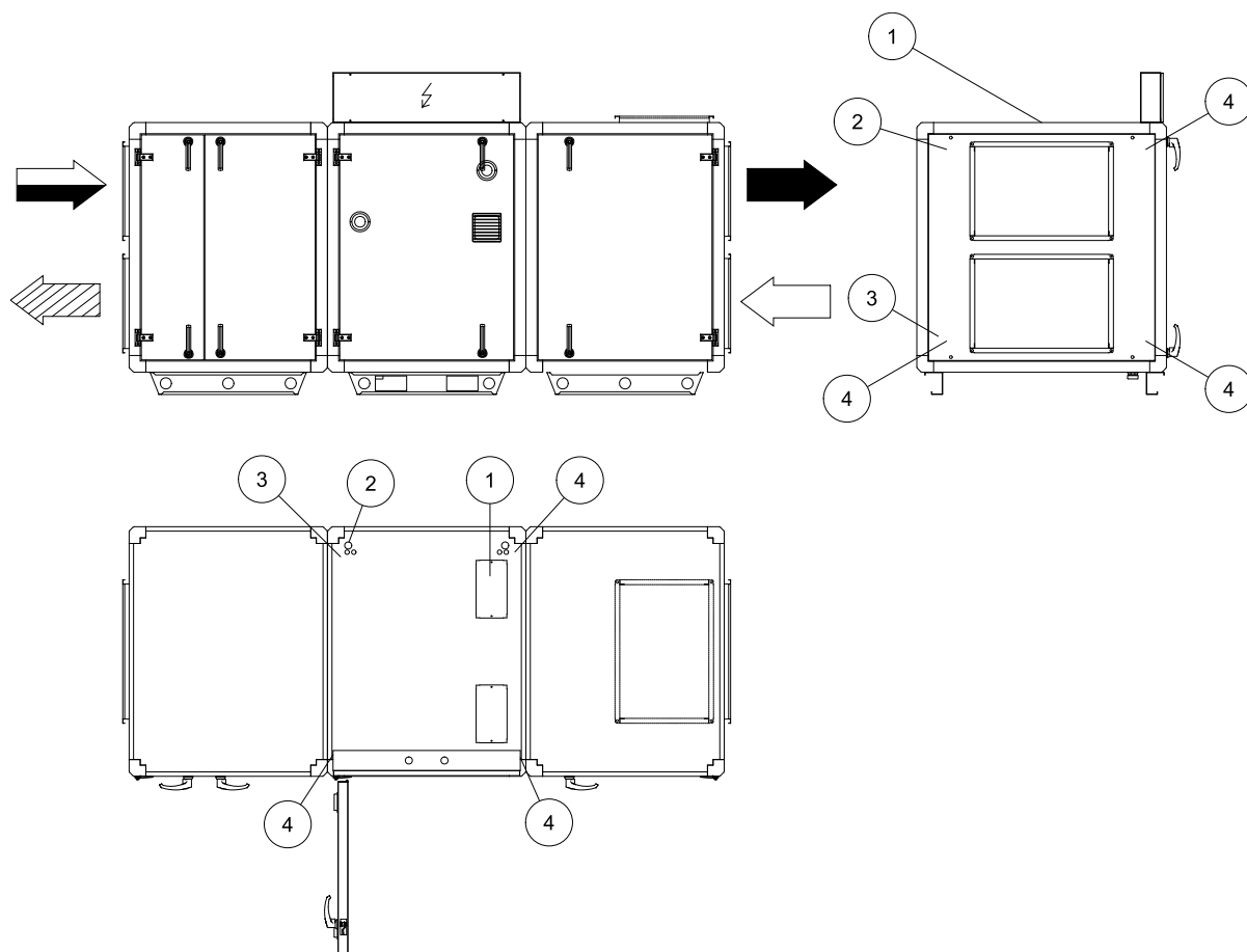
Рис. 6 Левосторонний агрегат (если используется правосторонний агрегат, нужно зеркально отобразить рисунок)
