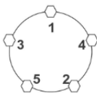
5-Lug Nuts
