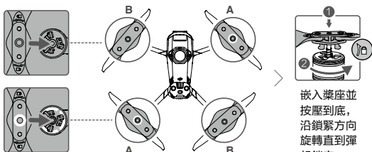
對準標記安裝螺旋槳
