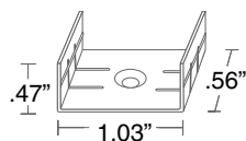
Plastic Clip (PLC-03)
