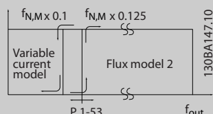
图 3.9 参数 1-00 配置模式 = [0] 开环速度, 参数 1-01 电动机控制原理 = [2] 无传感器矢量
