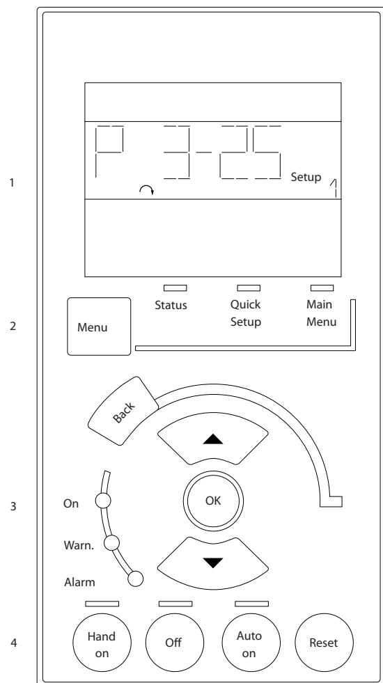
图 2.21 LCP 键
