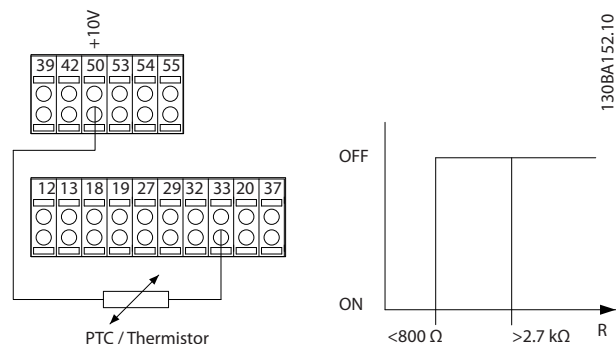
图 3.13 PTC 热敏电阻连接 - 数字输入
