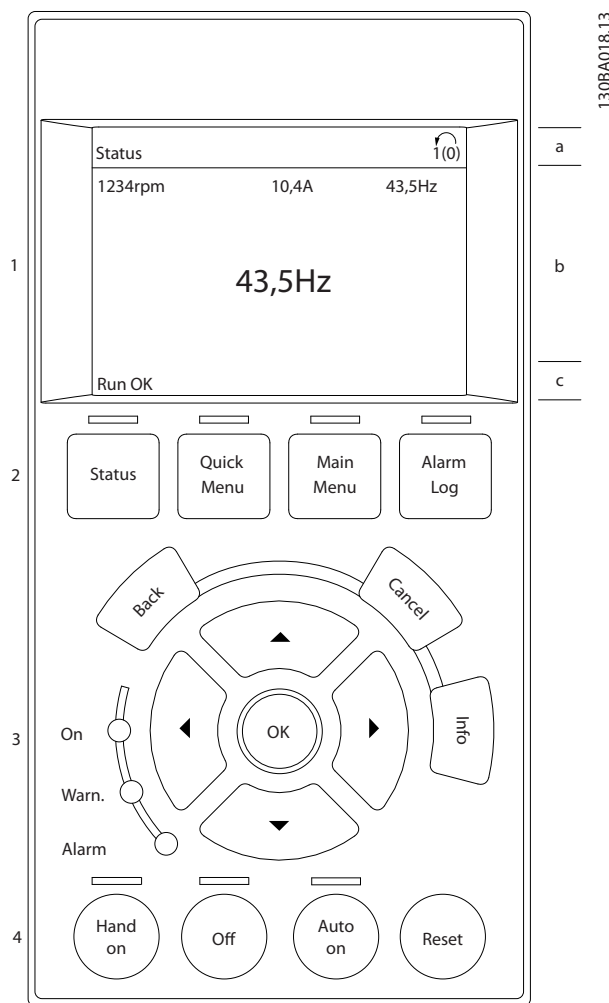
图 2.1 LCP
