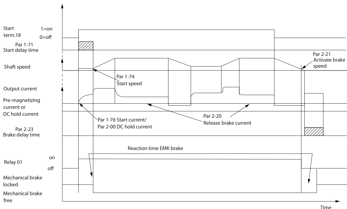
图 3.19 机械制动
