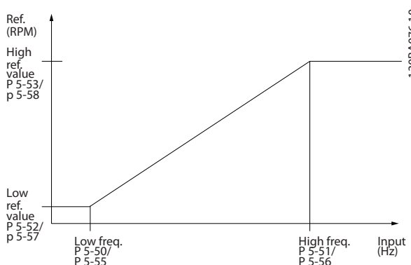
图 3.38 脉冲输入
