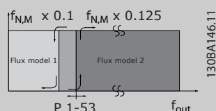
图 3.8 参数 1-00 配置模式 = [1] 闭环速度或 [2] 转矩和 参数 1-01 电动机控制原理 = [3] 磁通矢量带电动机反馈
