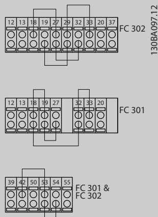
图 3.62 测试插头
