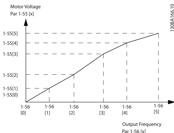
图 3.10 U/f 特性
