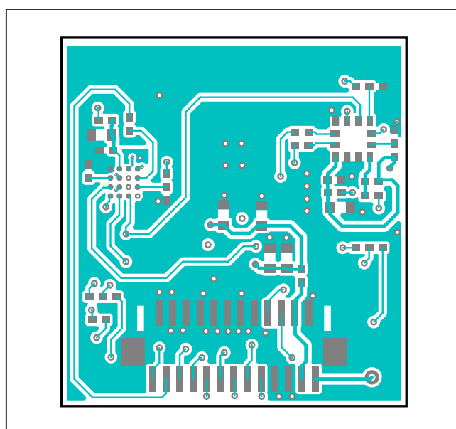
MAX86174A_OSB_EVKIT_B—Top Layer
