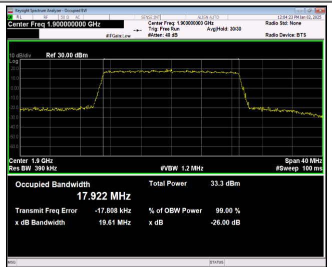
Band2-20MHz-16QAM-18900-100RB#0
