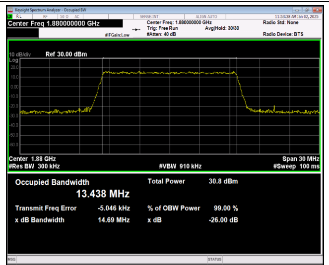
Band2-20MHz-QPSK-18700-100RB#0
