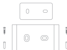
Wandhalterung (einschließlich Schraube 2, Wandstecker 2 und Montageschablonaufkleber)
