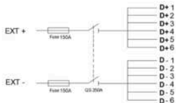
P-Combiner-HV-6
