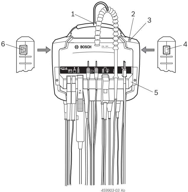
Sl. 1: FSA 500 sprijeda
