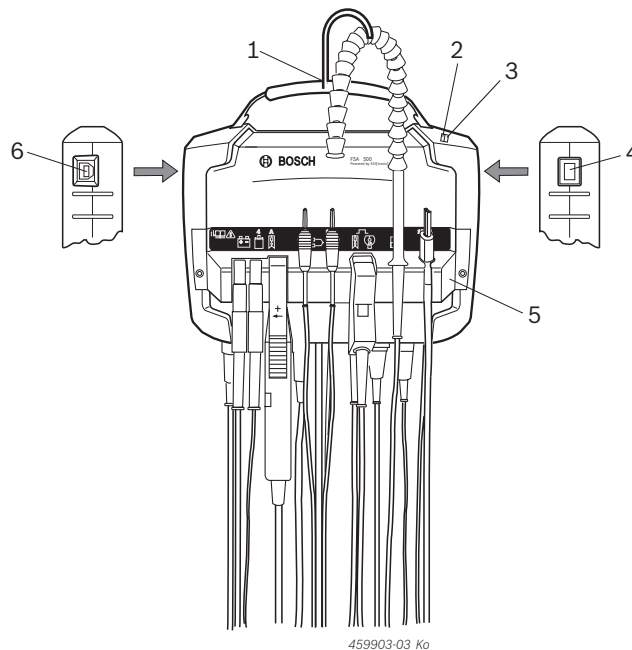
Abb. 1: Vorderansicht FSA 500
