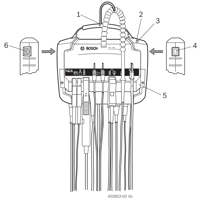
Afb. 1: Vooraanzicht FSA 500
