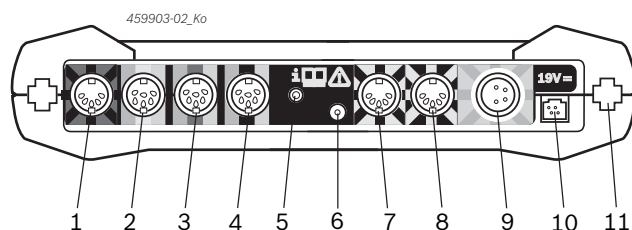
Kuva 2: Liitântälista FSA 500 (alhaalta)
