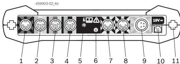
Sl. 2: Priključna letvica FSA 500 (odozdo)
