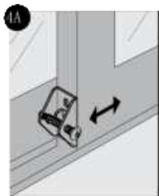
Grendelmontage op schuifdeur
