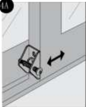
Zespół zatrzasku na drzwiach przesuwnych
