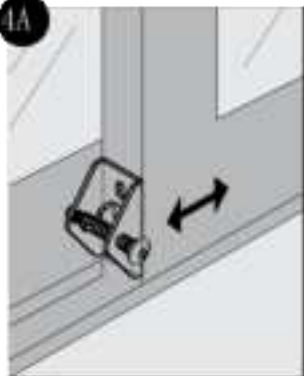
Riegelmontage an Schiebetür
