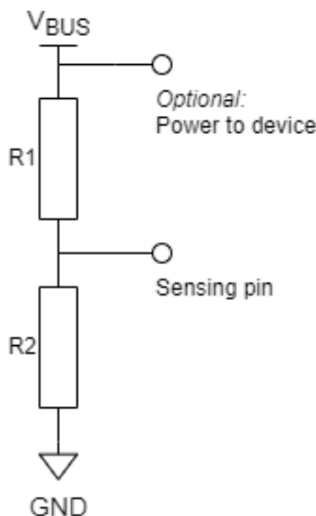
图 39: 用于 VBUS 监测的简易分压器
