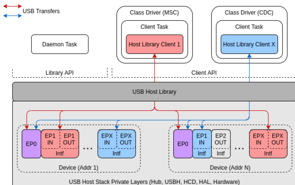
图 40: USB 主机功能涉及的关键实体
