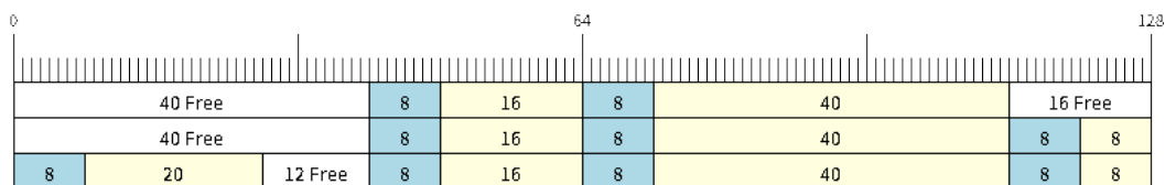
图 47: 在可分割 buffer 中绕回
