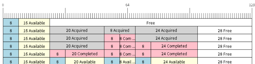
图 45: 在不可分割环形 buffer 中 SendAcquire/SendComplete 数据项
