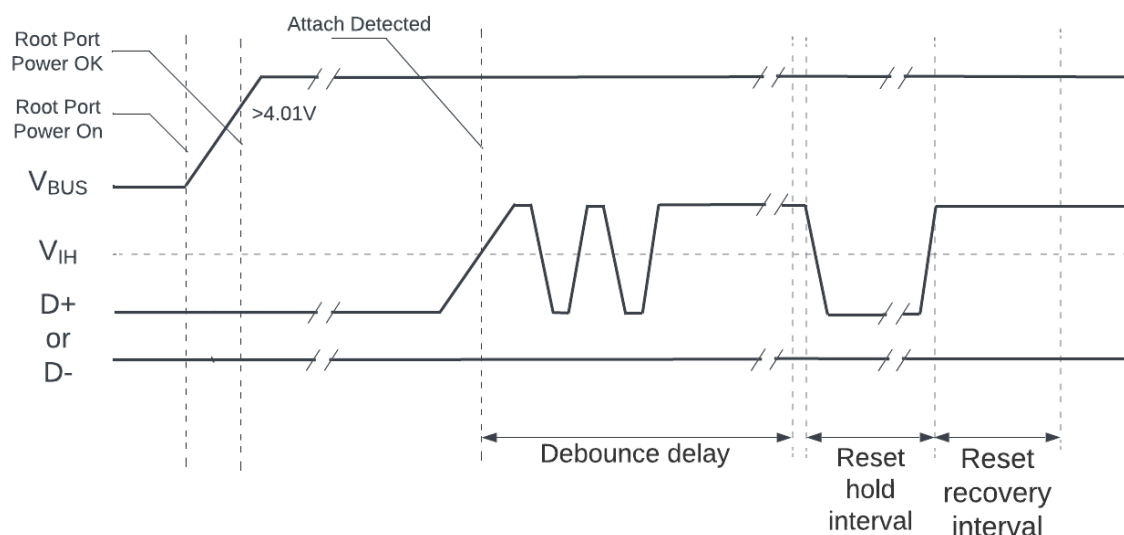
图 42: USB 根集线器上电和连接事件时序
