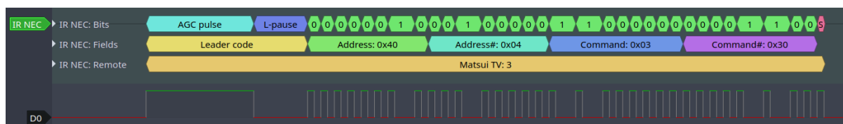
图 23: 红外 NEC 帧
