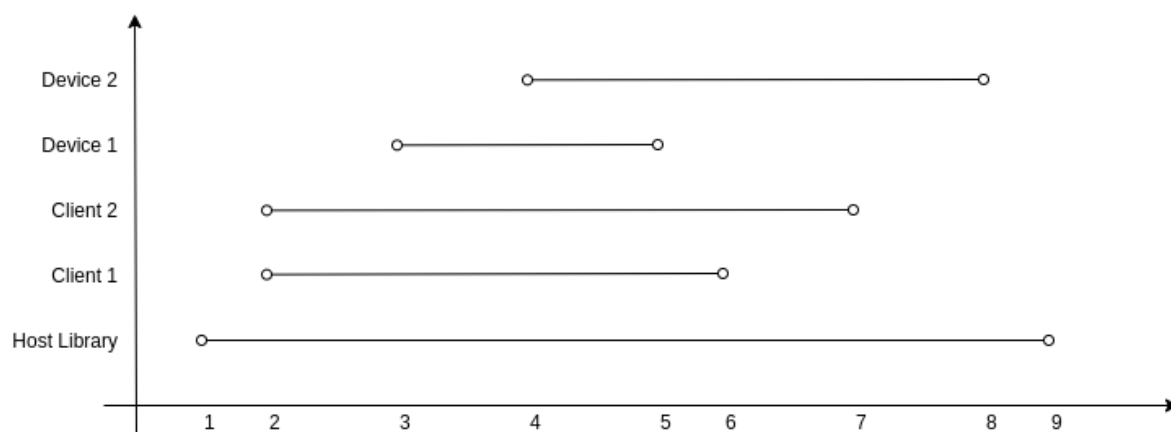
图 41: USB 主机库典型生命周期
