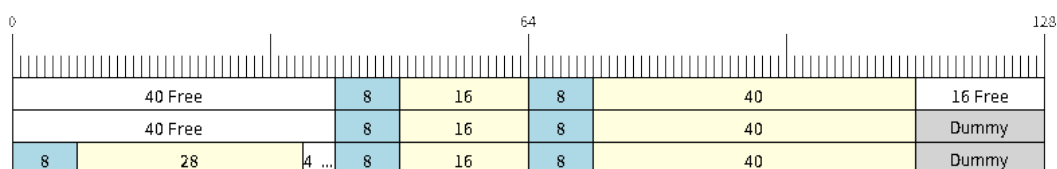
图 46: 在不可分割 buffer 中绕回
