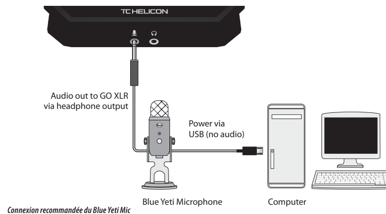
Connexion recommandée du Blue Yeti Mic
