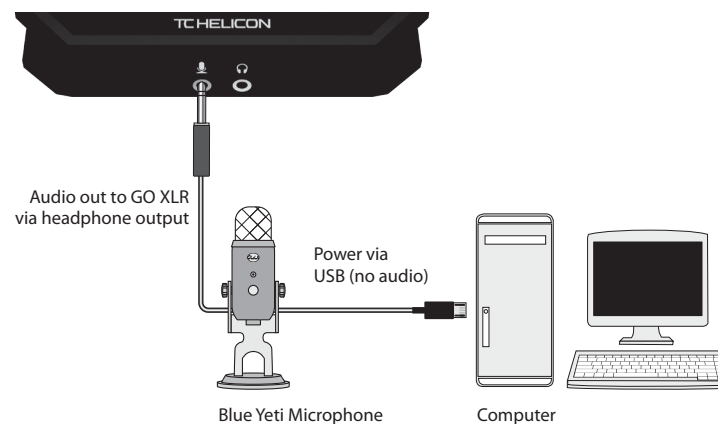
Conexão recomendada do Blue Yeti Mic
