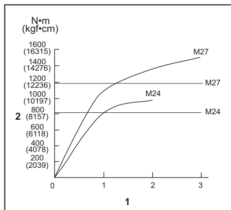
1. Tempo di serraggio (secondi) 2. Coppia di serraggio
