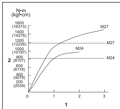
1. Tiempo de apriete (segundo) 2. Par de apriete
