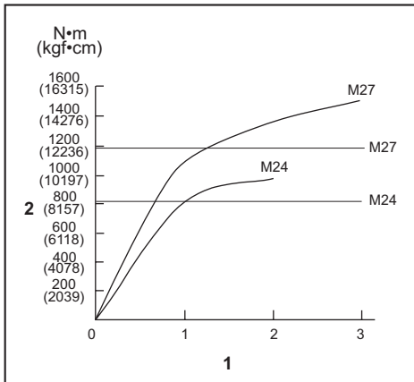
1. Anzugszeit (Sekunden) 2. Anzugsmoment
