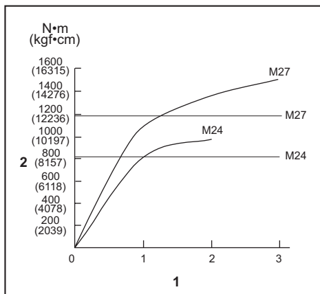
1. Tilspændingstid (sekunder) 2. Tilspændingsmoment
