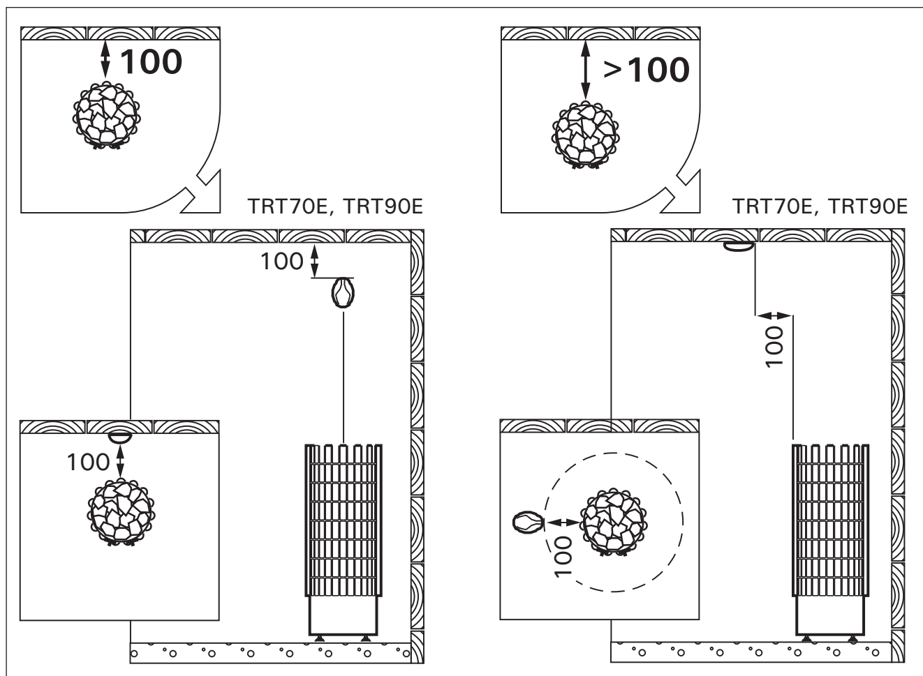
Kuva 8. Anturin asentaminen (mitat millimetreinä) Bild 8. Montering av givaren (mått i millimeter)
