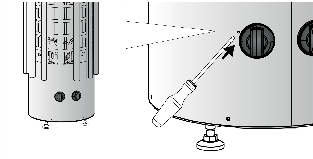
Kuva 10. Ylikuumenemissuojan palautuspainike
