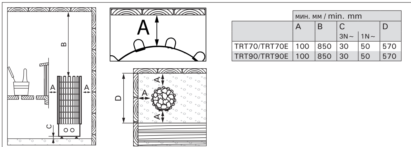
Рисунок 6. Расположение и безопасные расстояния (все размеры приведены в миллиметрах) Joonis 6. Ohutuskaugused (kõik mõõtmek millimeetrites)
