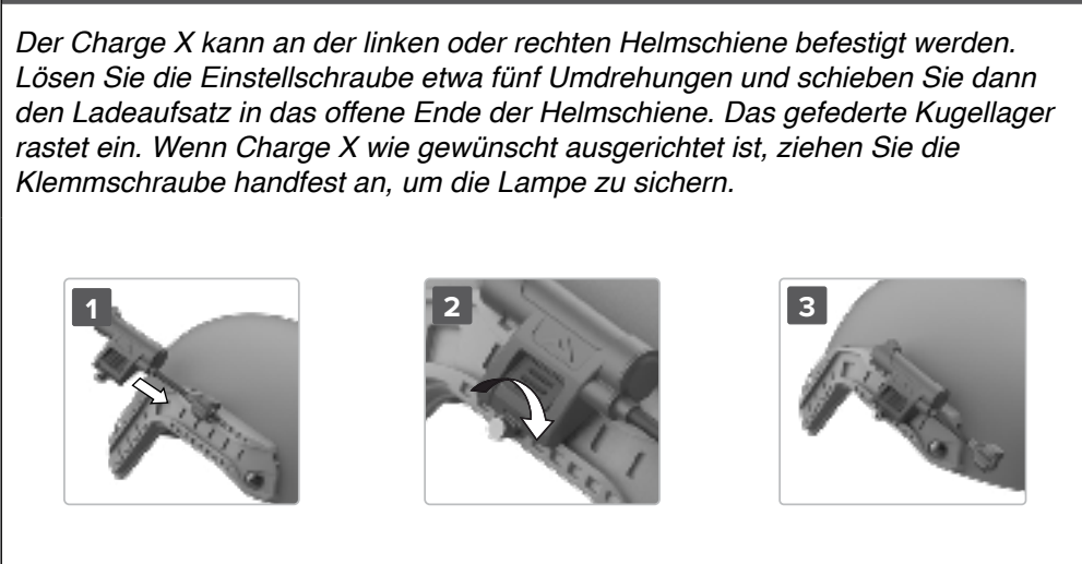
Abbildung 4 – Installation der ARC-Schiene
