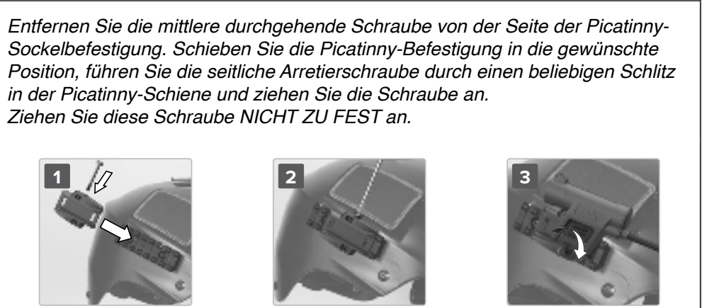
Abbildung 8 – Picatinny-Schienenbefestigung
