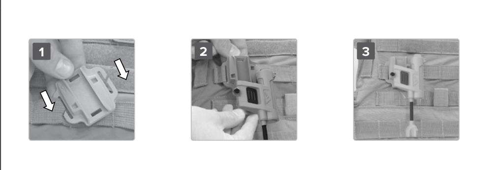
Abbildung 6 – M-LOK®-Befestigung
