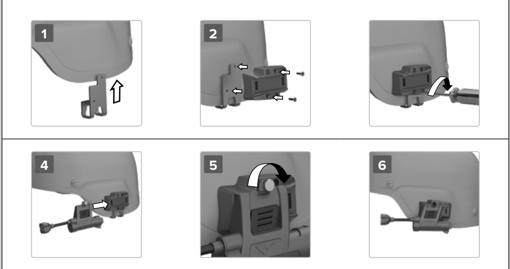
Abbildung 8 – Picatinny-Schienenbefestigung
