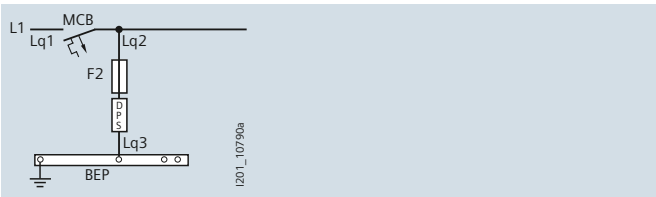
a) Proteção com MCB
