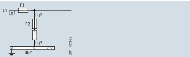
b) Proteção com fusível
