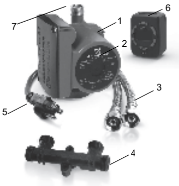
Fig. 10 Sistema Grundfos Comfort
