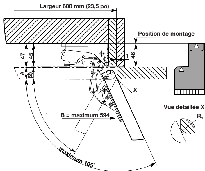
Épaisseur des murs de l'armoire de 16 mm
