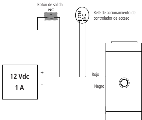
Esquema de conexión usando fuente del mercado
