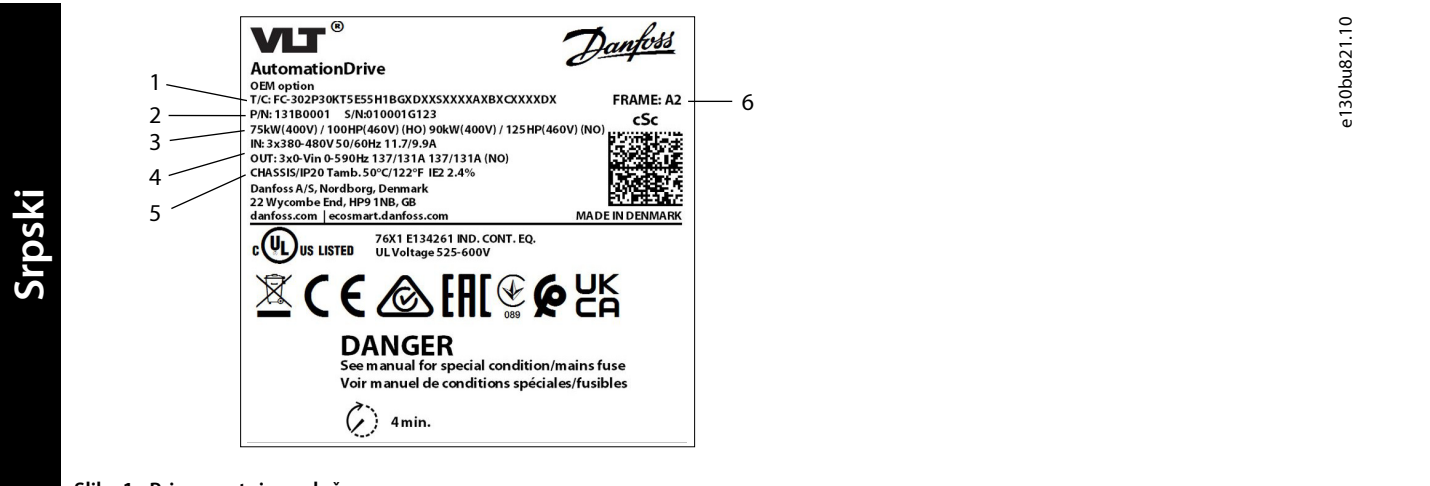
Slika 1: Primer natpisne ploče
