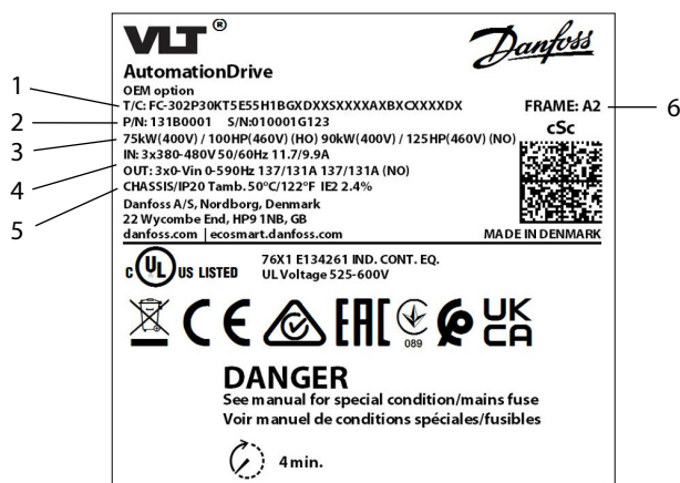
Obrázok 1: Príklad štítka výrobcu
