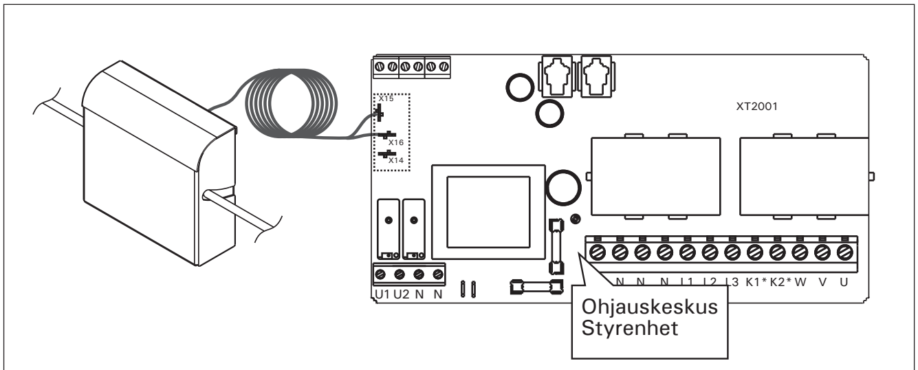
Kuva 4. Kytkentäkaavio Harvian ohjauskeskuksille Bild 4. Kopplingsschema för Harvias styrenheter
