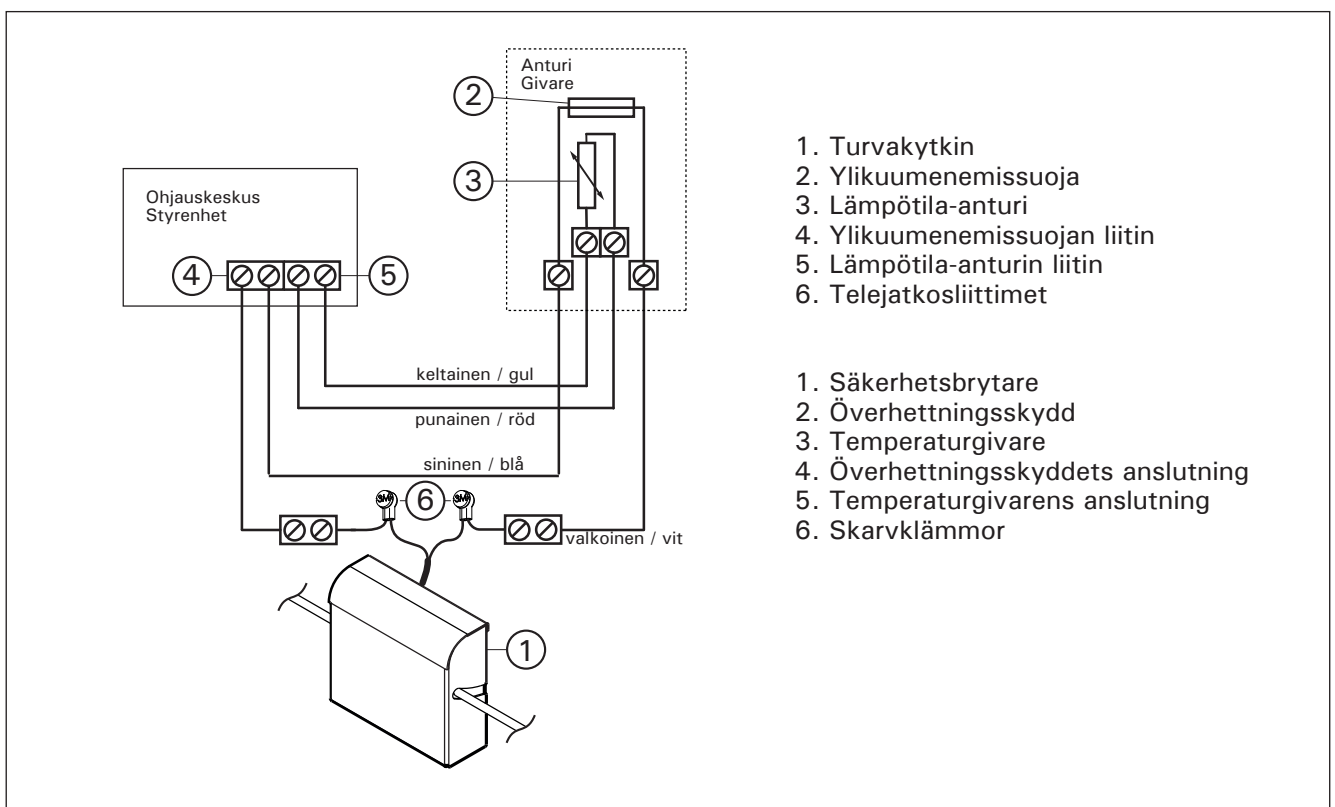
Kuva 5. KytKentäkaavio Sentiotec:n ohjauskeskuksille Bild 5. Kopplingsschema för Sentiotechs styrenheter
