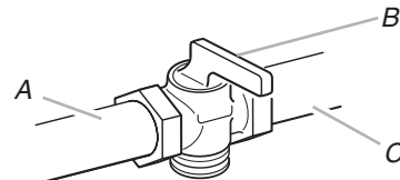
A. Canalisations de gaz B. Robinet d'arrêt en position « fermée » C. Vers la cuisinière
