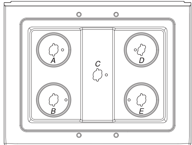
A. Standard burner - Natural gas orifice spud number 139
