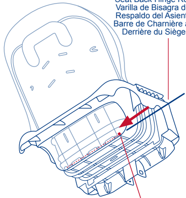
Fig. 2 Hinge rod retainer Sujetador de la vara de la bisagra Dispositif de retenue de la tige de support
