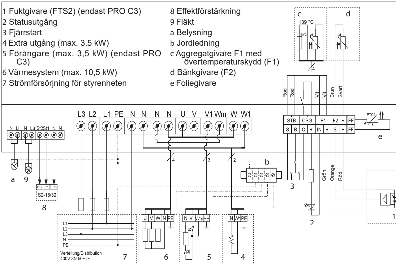
Bild4 Kopplingsschema
