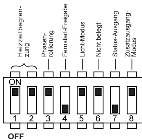
Abb.5 Funktionswahlschalter - Standardeinstellung
