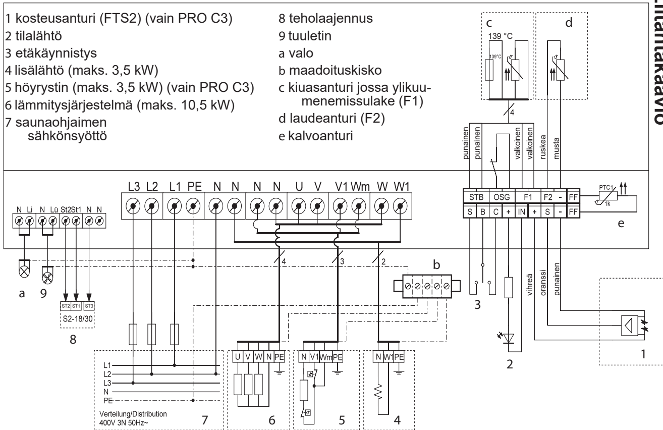
Kuva4 Liitântäkaavio
