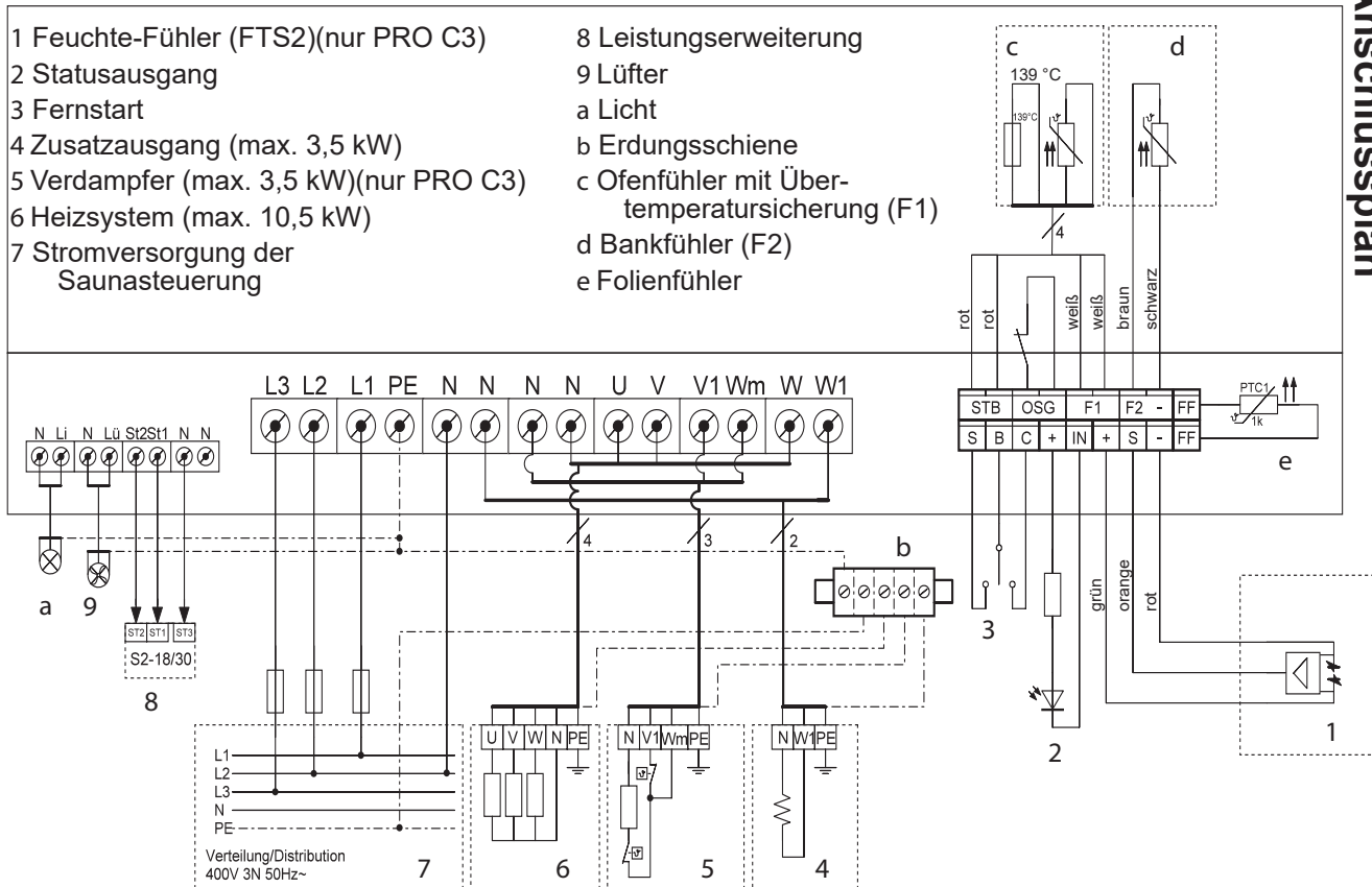
Abb.4 Anschlussplan
