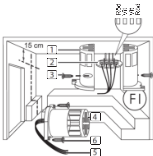
Bild3 Montering av urogivare
