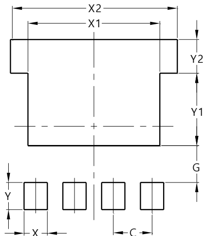
PowerDI8080-5
