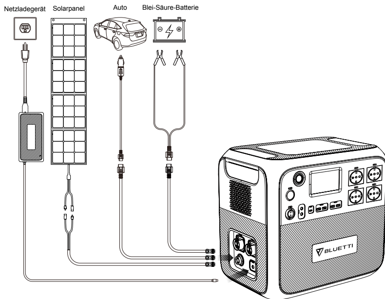
AC200MAX- Doppeltaufladungssystem
