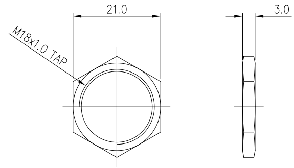
NUT
