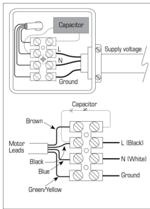
3 wire motor
