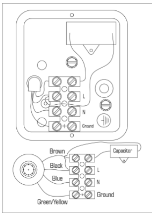
4 wire motor
