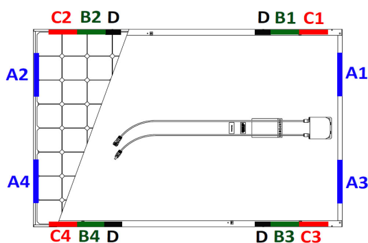
Figure 2 : Position des brides ou attaches de fixation pour les modules SunPower
