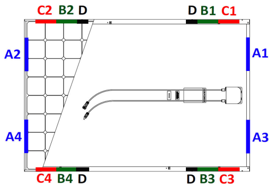
Abbildung 2: Befestigungszonen für Sunpower Module
