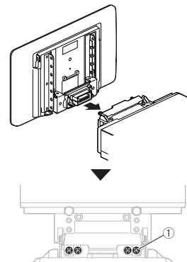
① Stelschroef (4 mm × 6 mm)
