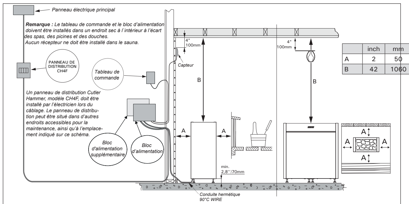
Figure 5. Commande du sauna / Distance de sécurité minimum / Installation du capteur
