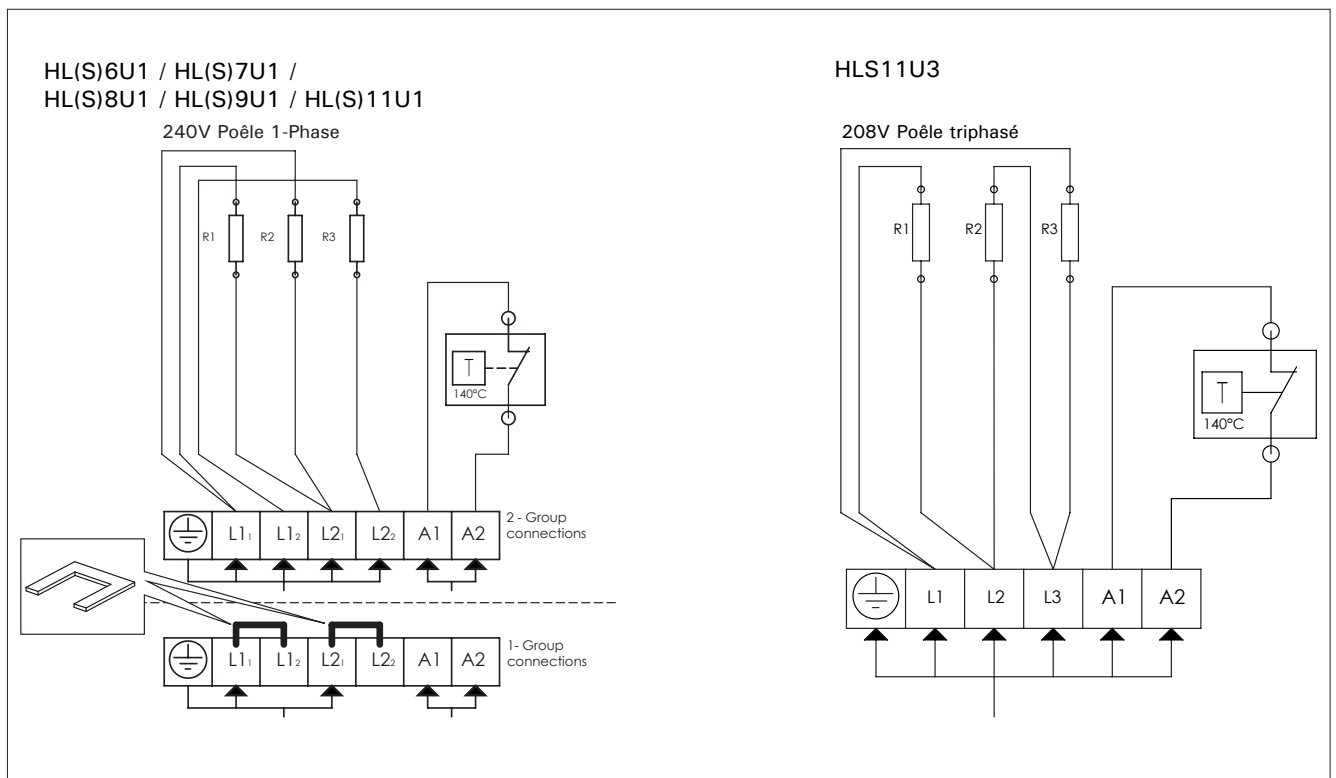
Figure 6. Connexions électriques du poêle
