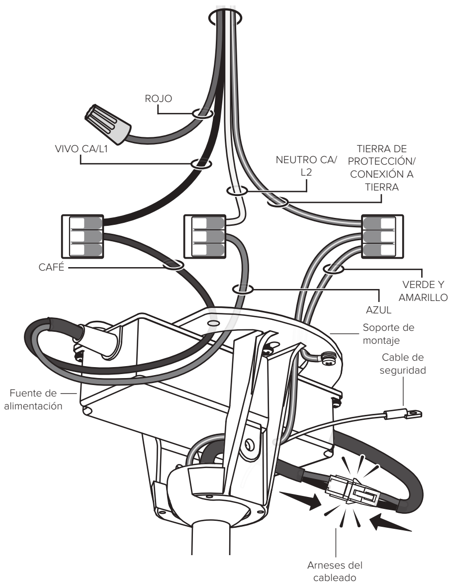
Fig. 11a: Diagrama de cableado (sin filtro EMI)
