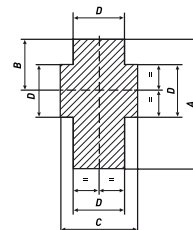
Fig. 2 — Dimensions minimum des zones protégées
