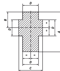
Bild 2 — Skyddszonernas minimimått
