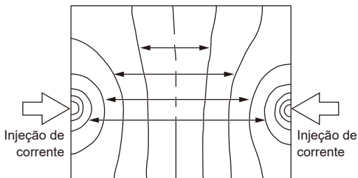
Figura 1: As linhas equipotenciais em uma placa de metal, mostrando a distribuição da corrente em intervalos de 50\ \mu\text{V} quando uma corrente de 1\ \text{A} é aplicada nos pontos distais da placa ( L300 \times C370 \times e0,4 )
