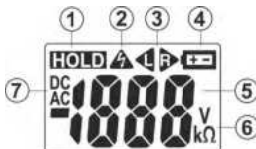
Fig. 3: Descrizione display LCD
