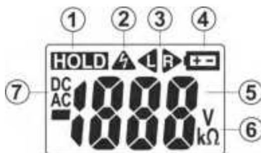
Fig. 3: Description de l'afficheur LCD
