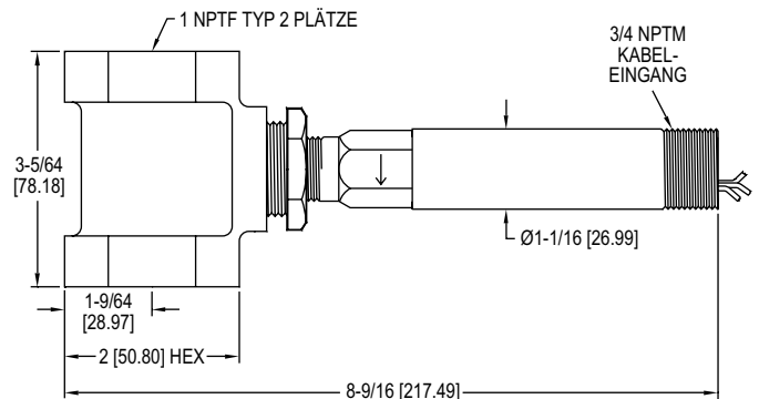
Mit T-Stück
