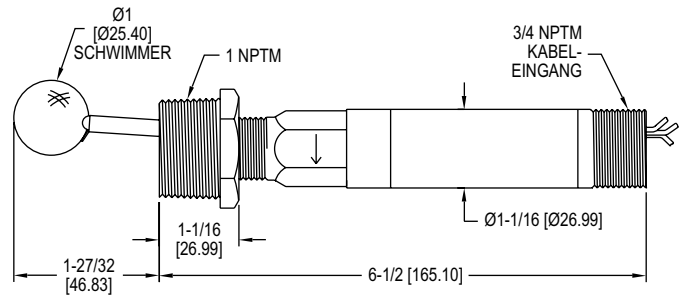
Runder Edelstahlschwimmer
