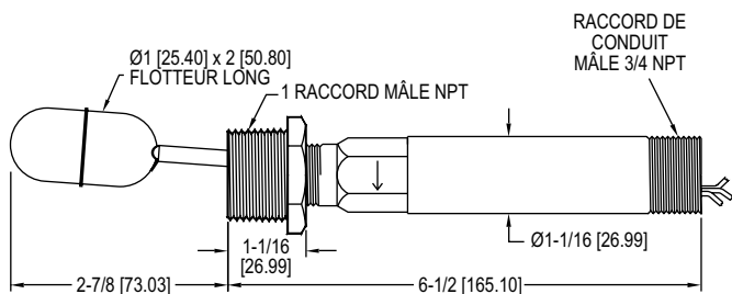
Flotteur cylindrique en acier inox
