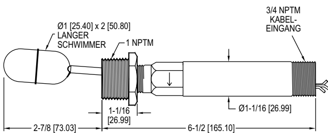
Zylindrischer Edelstahlschwimmer
