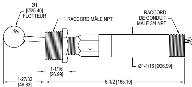
Flotteur rond en acier inox
