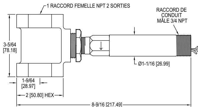
Avec chambre externe à flotteur (té)
