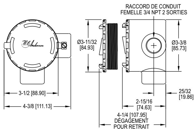
boîtier CSA, IECEx, ATEX
