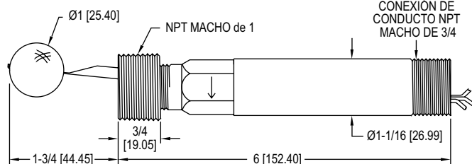
Flotador de polipropileno
