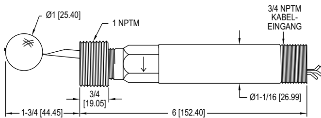
Polypropylenschwimmer
