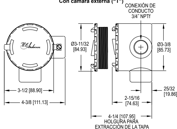
CSA, IECEx, caja del conductor ATEX
