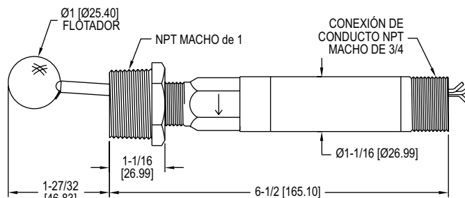
Flotador esférico de acero inoxidable
