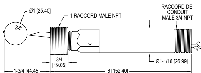
Flotteur en polypropylène
