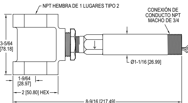
Con cámara externa ("T")
