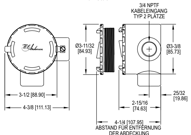
IECEx, ATEX-Gehäuse
