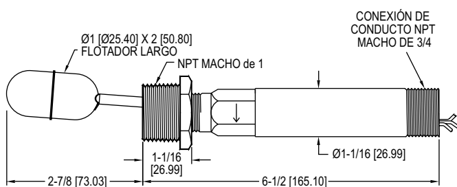
Flotador cilíndrico de acero inoxidable
