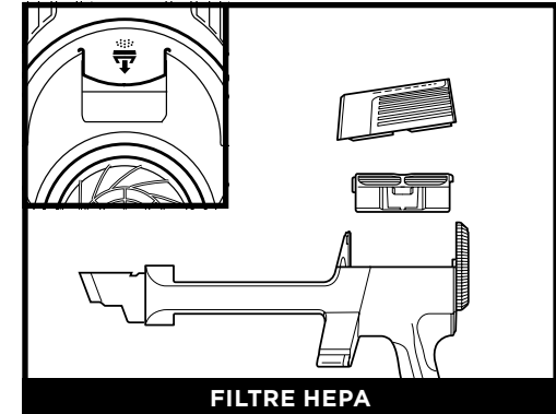
FILTRE HEPA
