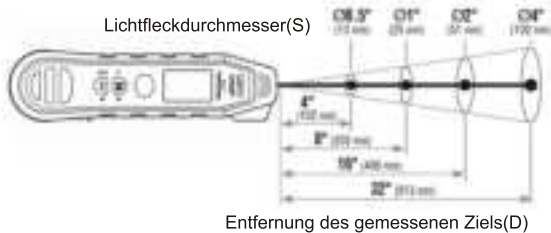
Der Lichtfleckdurchmesser repräsentiert 95 % der Energie
