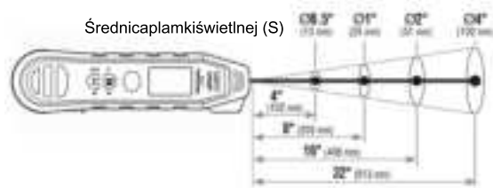
Odległość mierzonego celu (D)
