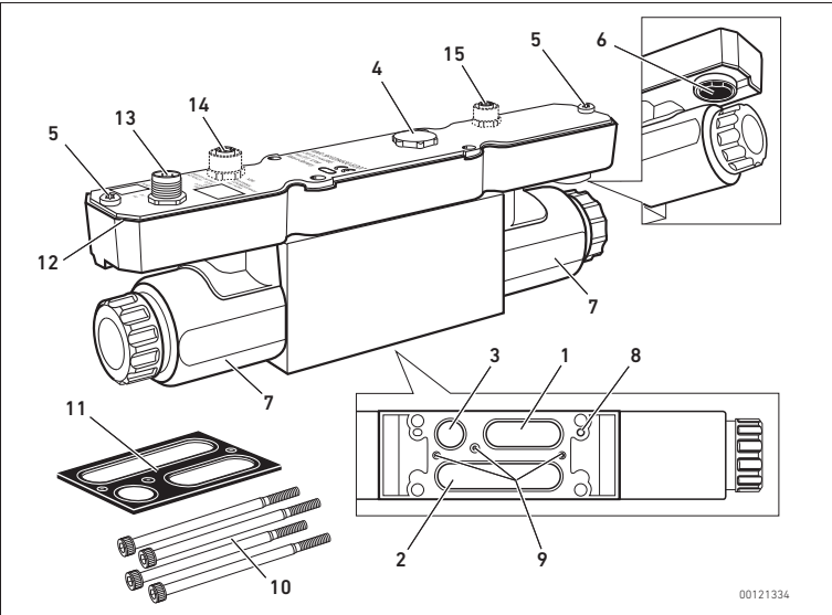
Fig. 1: V lvula reguladora de presi n ED07
