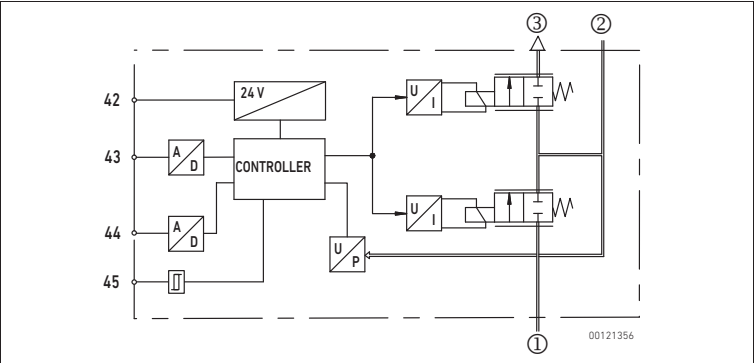
Fig. 4: Schéma fonctionnel
