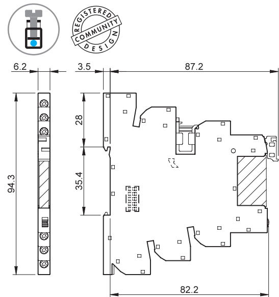
Types 39.80 39.81 Bornes à cage
