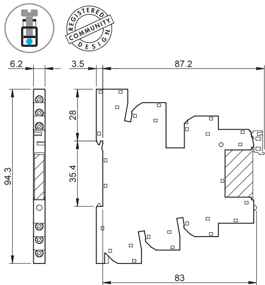
Types 39.40 39.41 Bornes à cage
