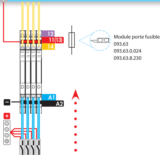
Dispositif en entrée d'automate
