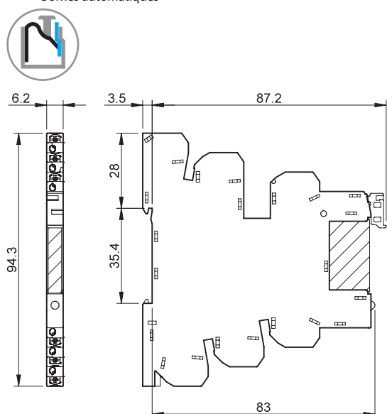
Types 39.70 39.71 Bornes automatiques
