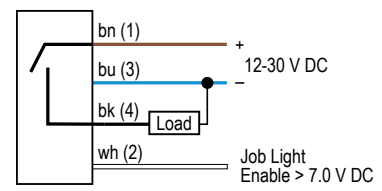
PNP 型号
