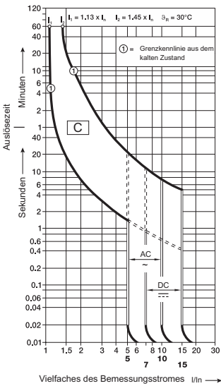
Auslösecharakteristik C
