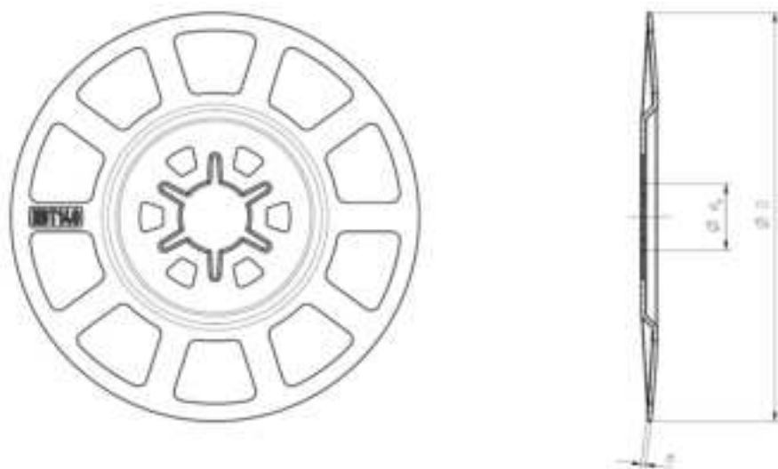
Rysunek A5: Opcjonalny talerzyk dociskowy HDT 140
