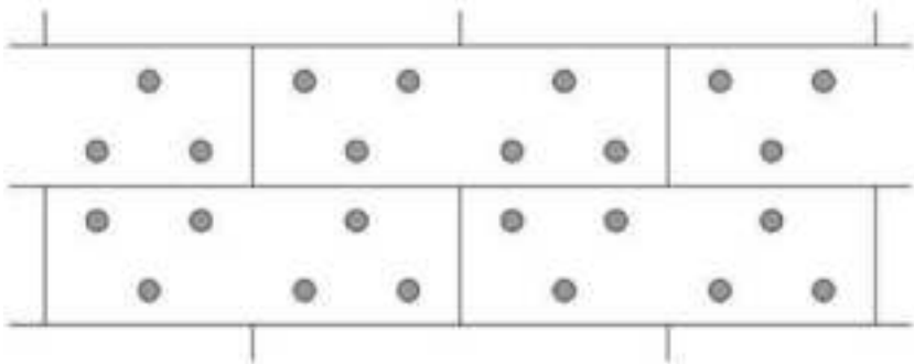
Rysunek B1: Układ kotew w przypadku zastosowań stropowych
