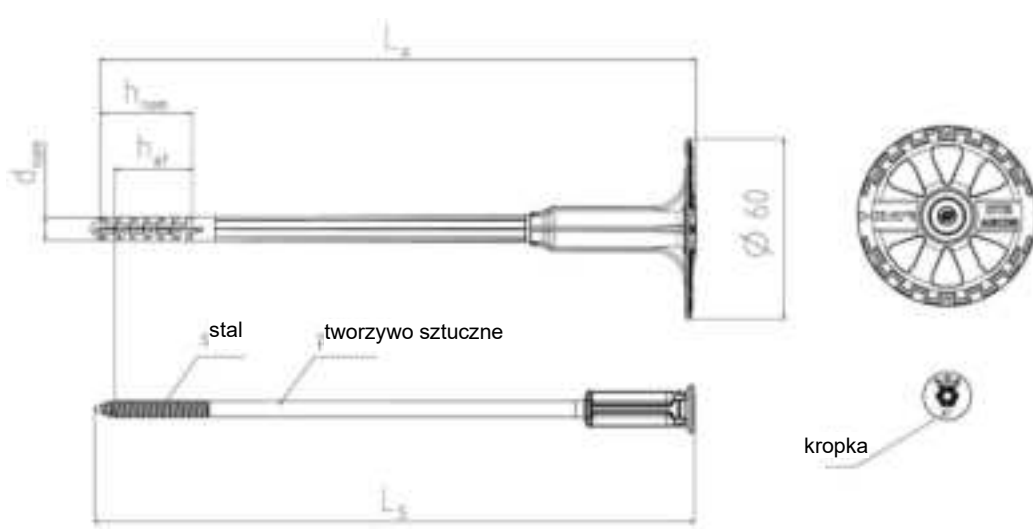
Rysunek A2: HTR-M - zamontowana tuleja, talerzyk dociskowy i śruba kompozytowa
