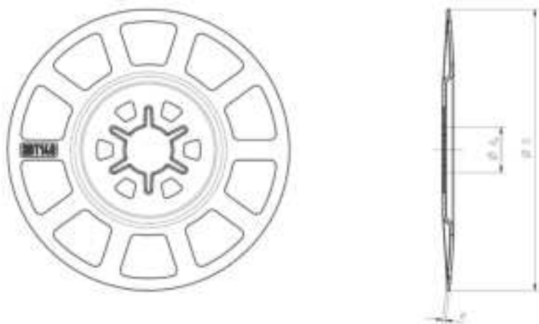
Abbildung A5: Zusatzsteller HDT 140
