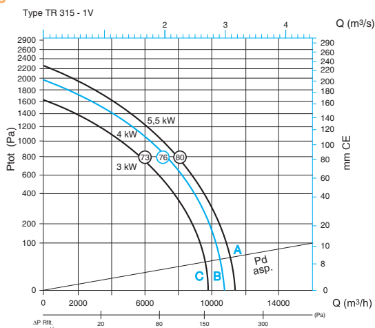
Caractéristiques aérodynamiques ProtectONE® TR 315 - 1V
