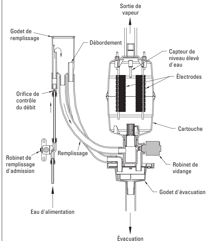
FIGURE 1 – Système de remplissage et d'évacuation et cartouche
